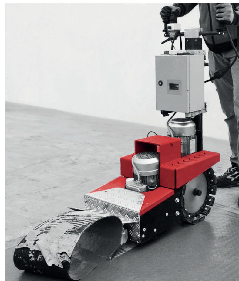
Rimozione linoleum con MAXISTRIPPER 200
