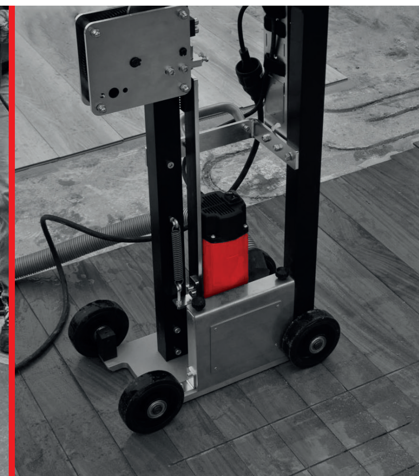
Pre-taglio parquet con MAXIPRECUT 180
